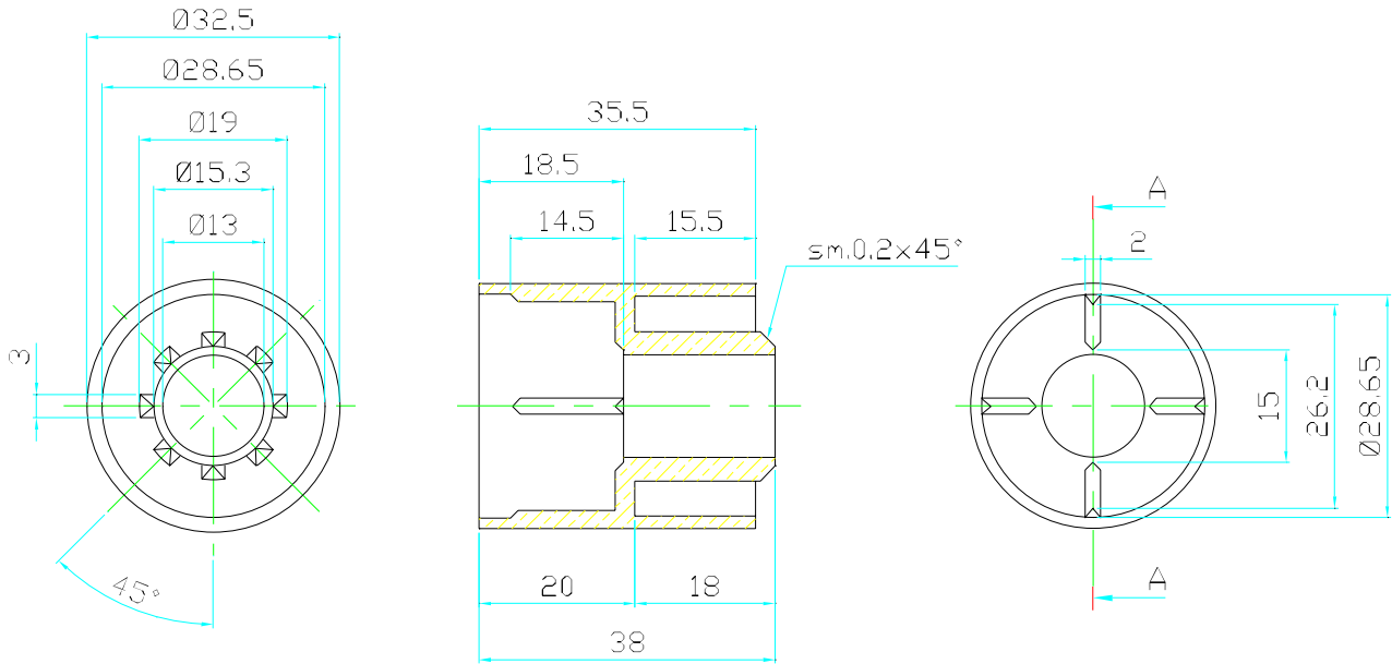
Sez. A-A
