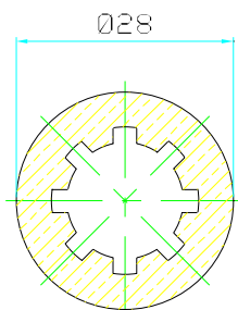
Sez. A-A
