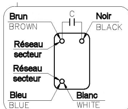
Pompe avec marche à gauche en regardant sur l'arbre
