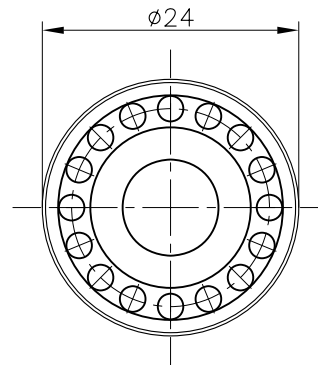
24-S w.st.nr: 1.4122 Gehärtet 42 Rc
