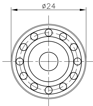
24-AS w.st.nr: 1.4122 Gehärtet 42 Rc
