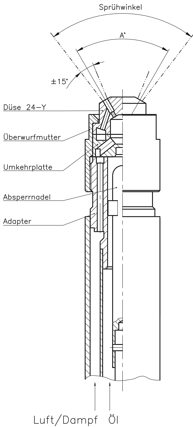
Nadel geöffnet
