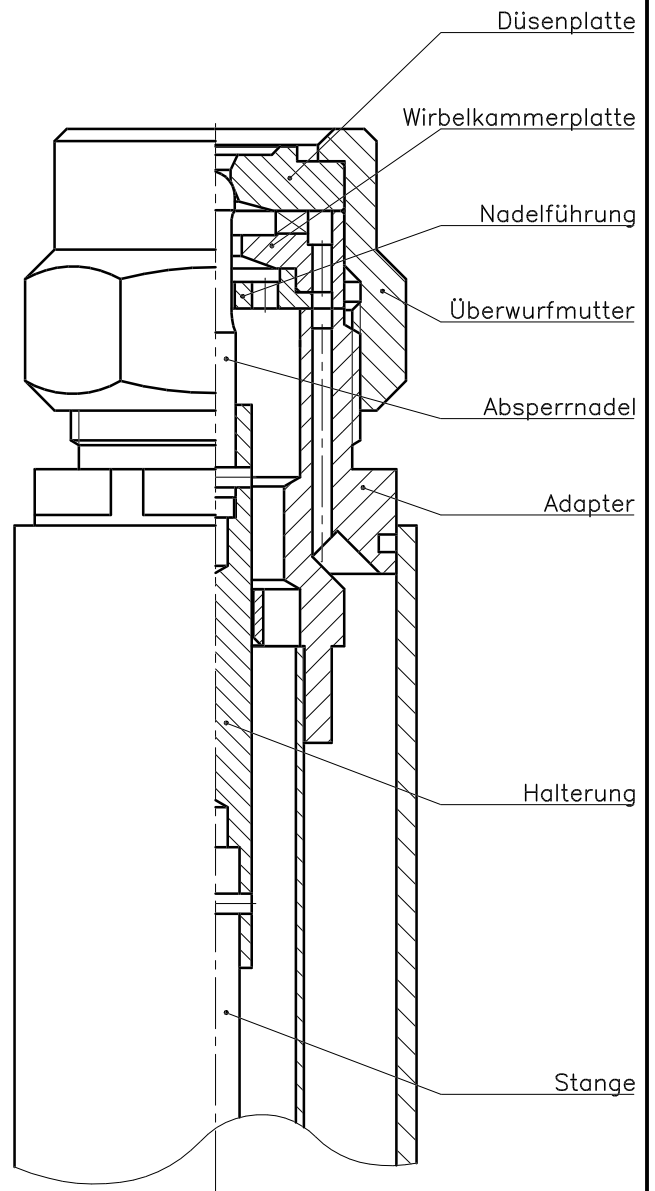
Nadel geschlossen
