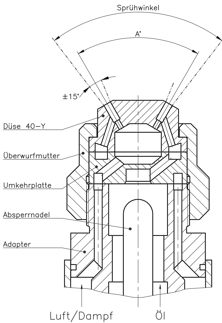
Nadel geöffnet
