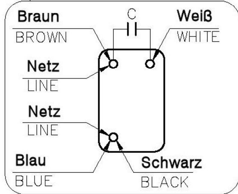
Drehrichtung links auf Motorwelle gesehen
