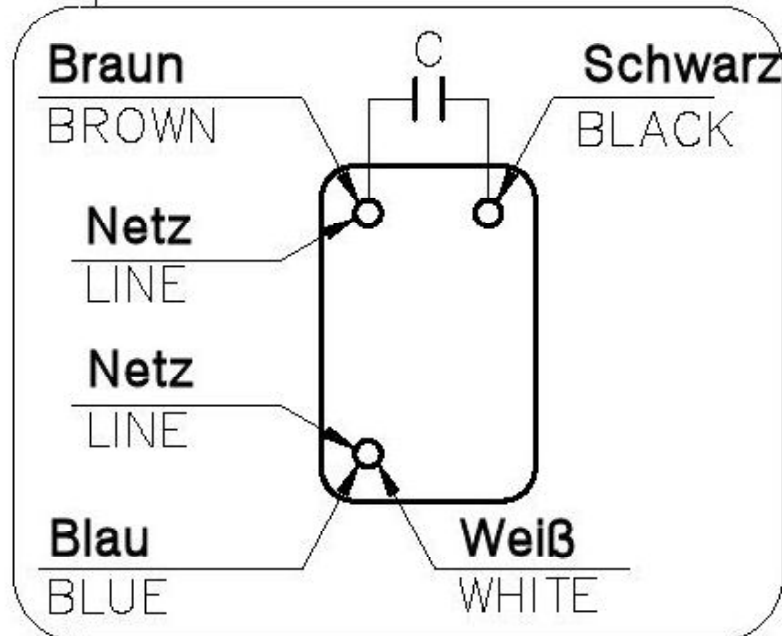
Drehrichtung rechts auf Motorwelle gesehen
